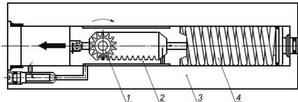
б) закрывание двери
