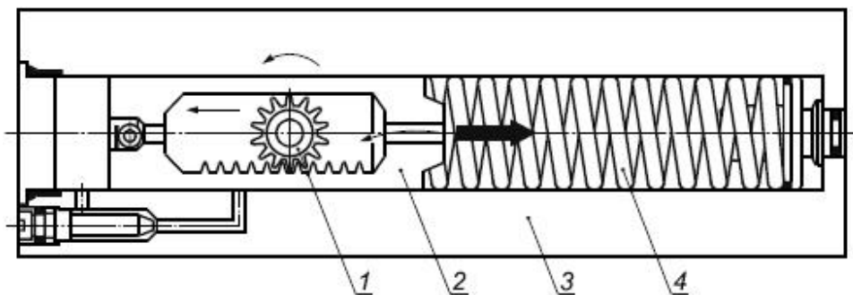
а) открывание двери
